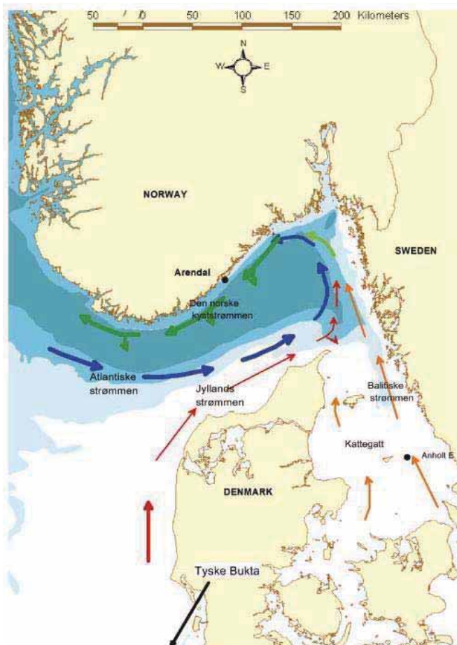
Figur 7. Skjematisk strømkart for Skagerrak.
