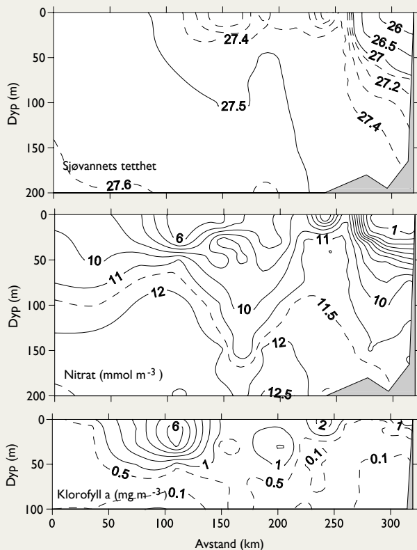
Figur 7. Svinøysnittet. Vertikal fordeling av vannets tetthet og nitrat i de øverste 200 meterne og klorofyll a i de øverste 100 meterne i første uke av mai 2010. Svinøy section. Vertical distribution of water density and nitrate in the upper 200 meters and chlorophyll a in the upper 100 meters during the first week of May 2010.
