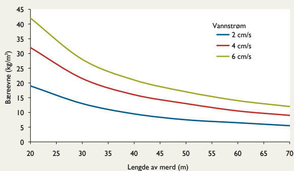
Figur 2. Beregnet midlere bæreevne som tetthet ( \text{kg}/\text{m}^3 ) ved ulike lengder av merden og vannstrøm 2, 4 og 6 cm/s gitt normal sommertemperatur og oksygennivå (sjøvann, 15 °C, 9,5 mg/l, 115 % metning). Laveste akseptable gjennomsnittlige oksygenverdi i merden er satt til 7 mg/l (85 % oksygenmetning).
