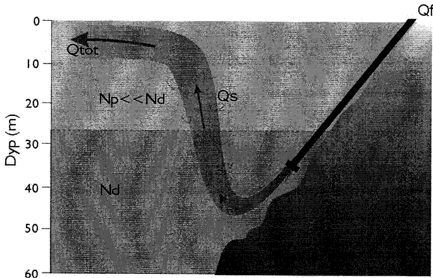
Fig. 14. Prinsippsskisse for kunstig oppstrømning av dypvann ( Q_{tot} = Q_f + Q_s ) ved dykket ferskvannsutslipp ( Q_f ). Q_s = tilført dypvann. N_d = næringsalter dypvann og N_p = næringsalter i produksjonslaget etter vårblomstring.
